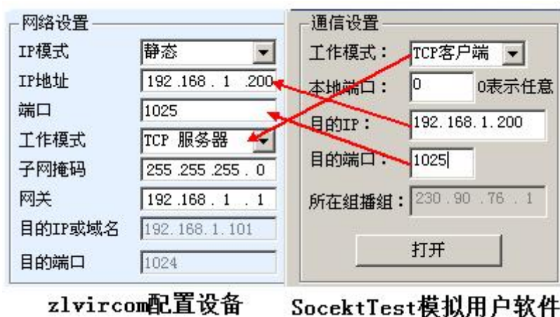
图 21 串口服务器作为服务端
