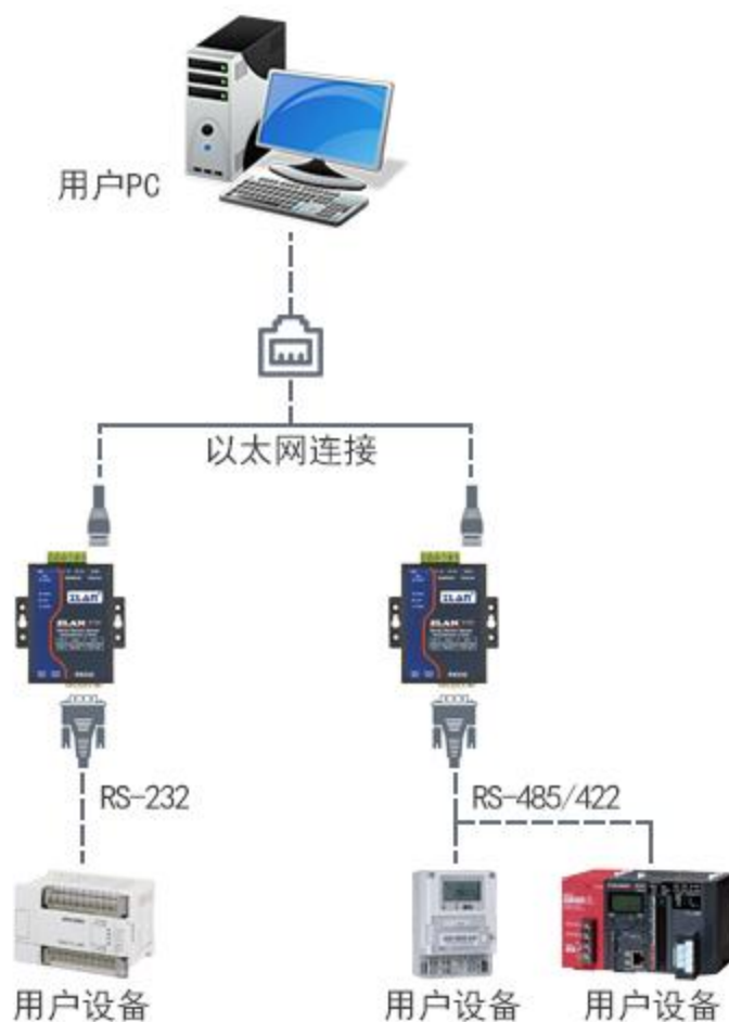
图 3 连接示意图
