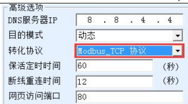
图 18 启用 Modbus TCP 功能
