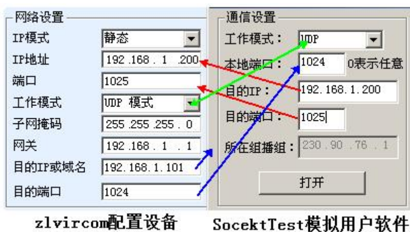
图 22 UDP 模式参数配置
