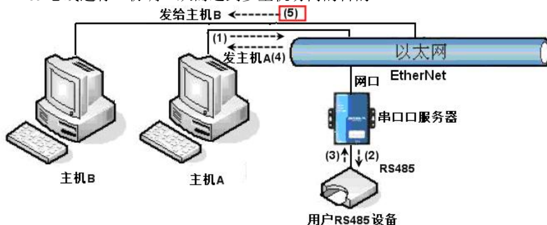
图 31 多主机功能演示
