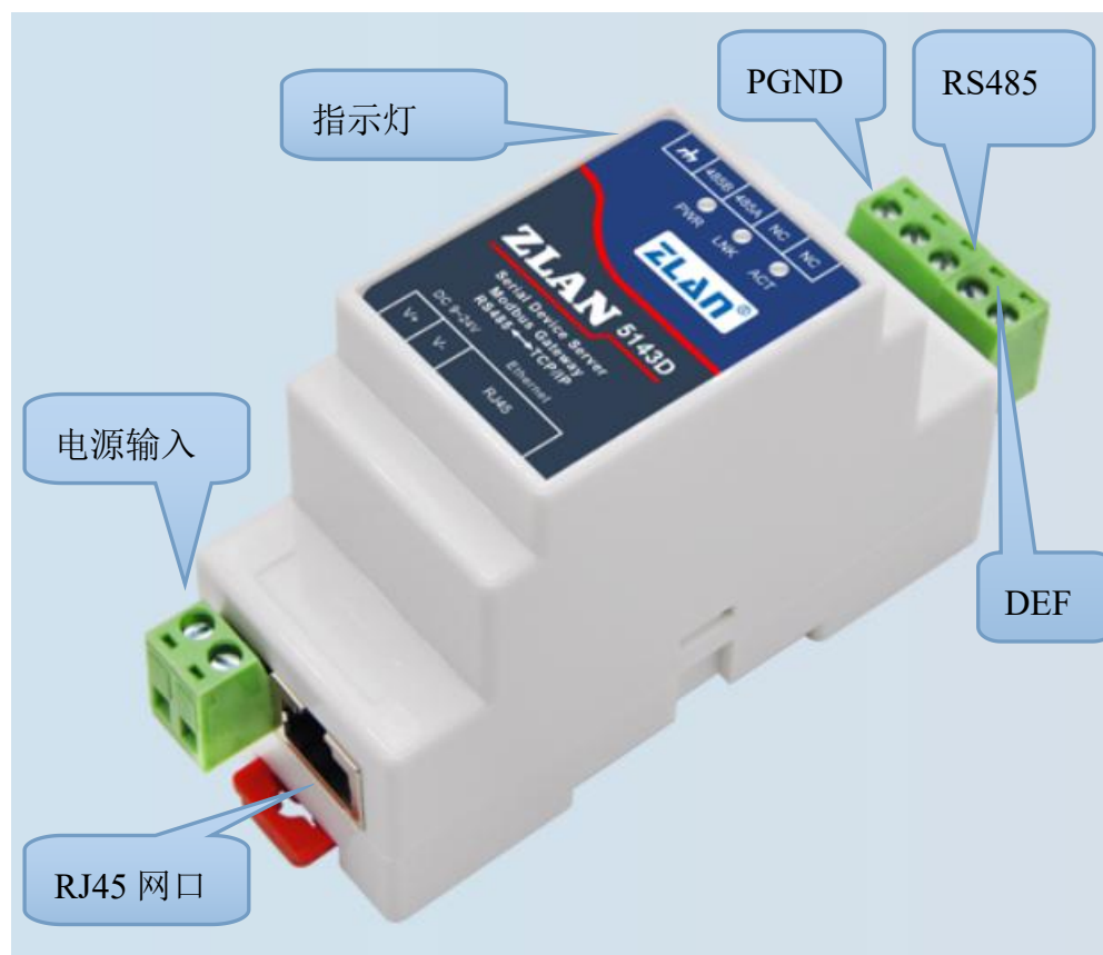
图 4 正视图
