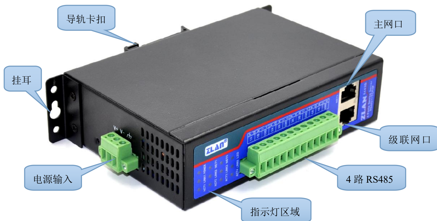
图 3 正视图
