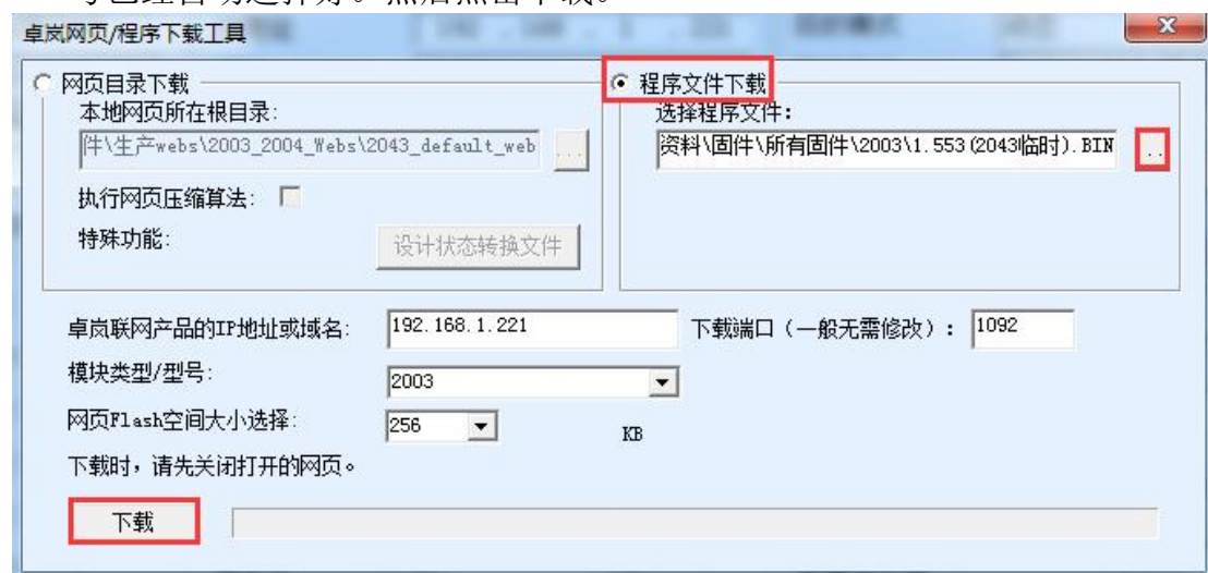
图 49 ZLSN2003 固件升级方法
