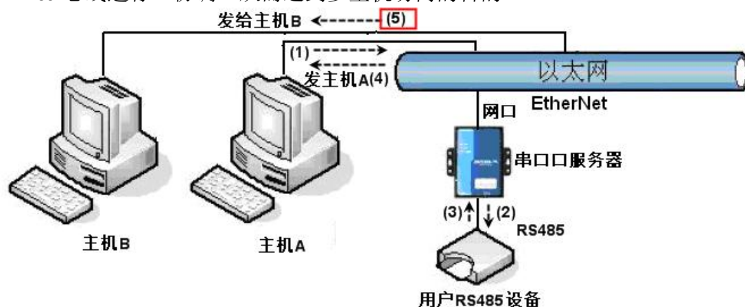
图 35 多主机功能演示
