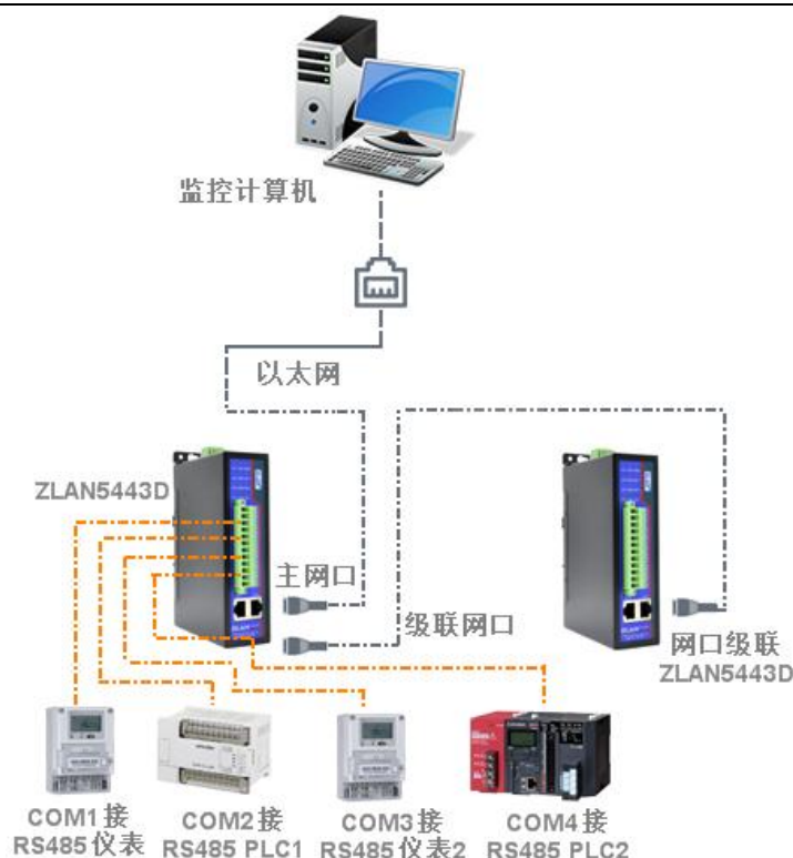
图 2 连接示意图
