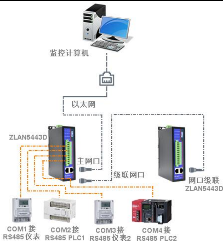
图 2 连接示意图
