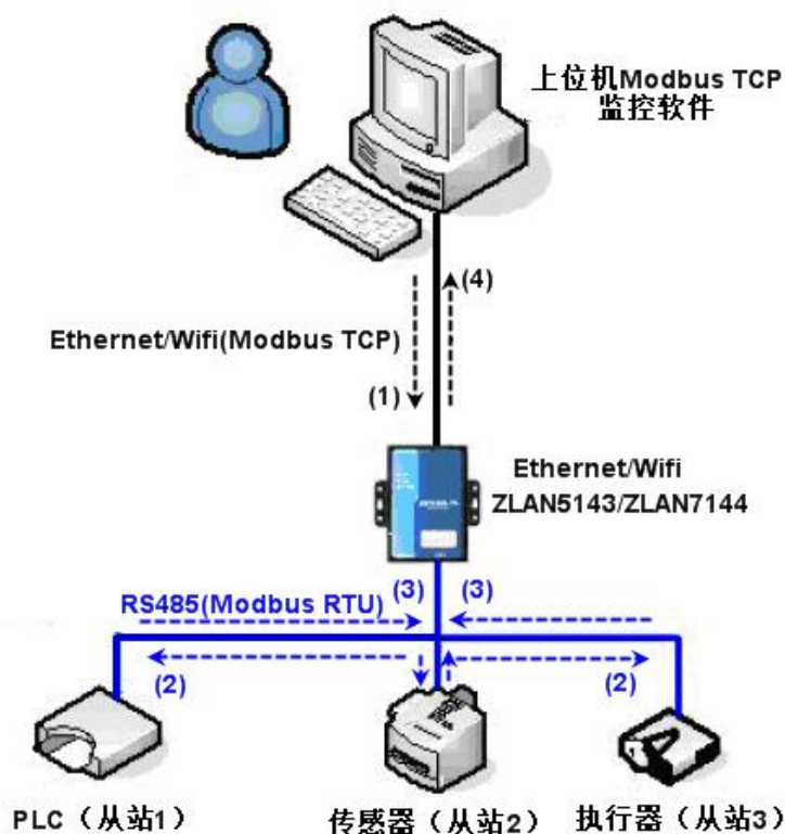
图 33 存储型 Modbus 网关工作方式
