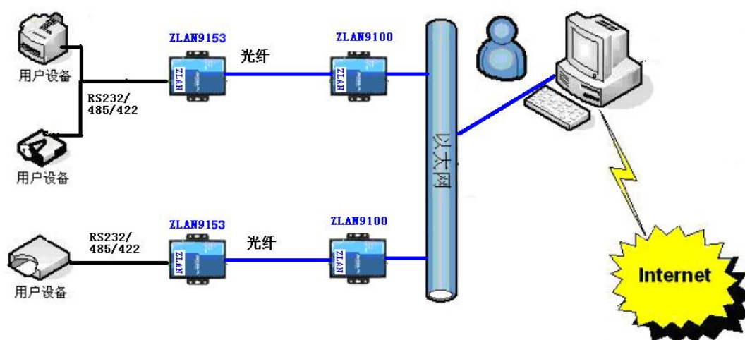
图 2 连接示意图
