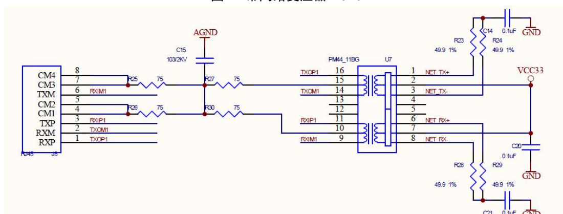
图 8 RJ45 和网络变压器分开方式
