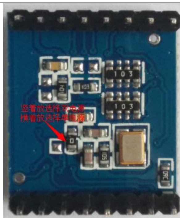
图 5 双电源和单电源模块差别
