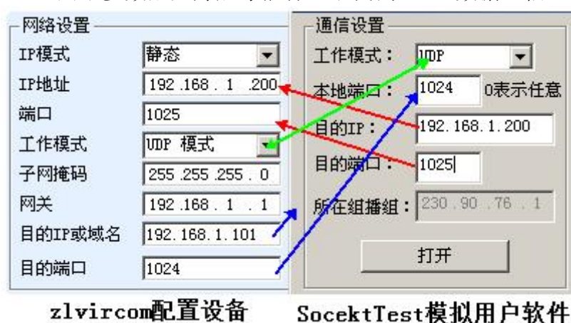
图 31 UDP 模式参数配置
