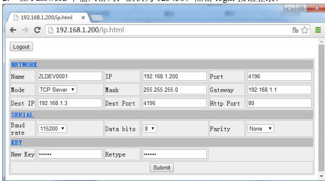
图 25 Web 配置界面
