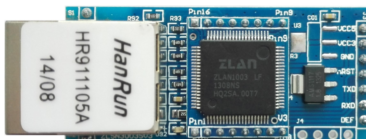
图 9 ZLSN3003S 外观图
