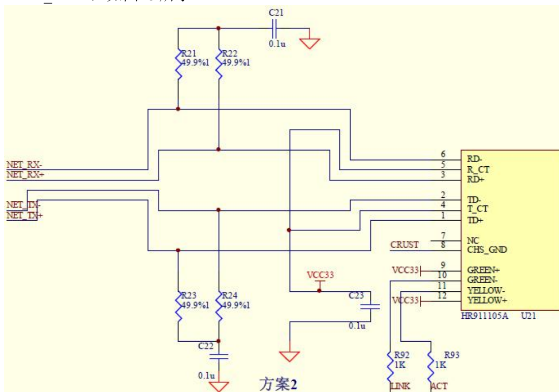
图 7 带网络变压器 RJ45
