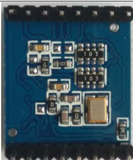
图 2 ZLSN2003S 背面图
