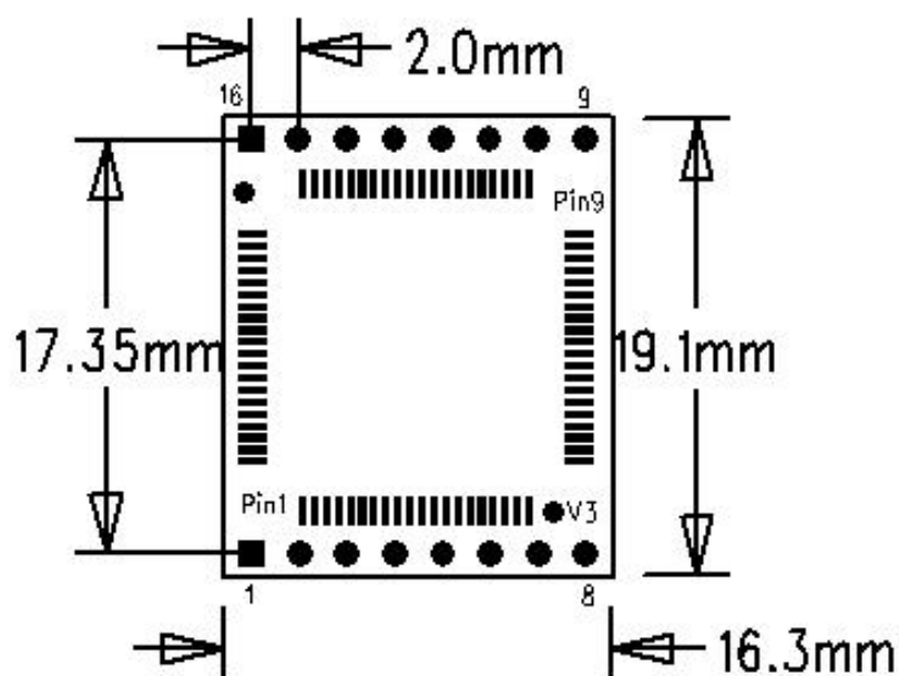
图 4 ZLSN2003S 正面引脚图
